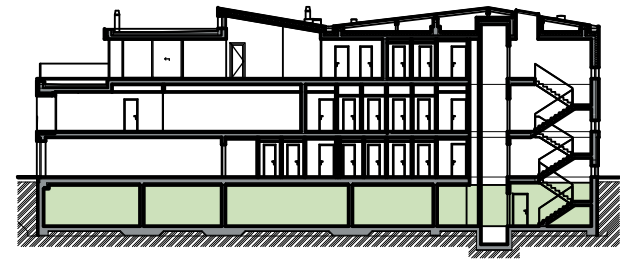
SCHEMATICKÝ ŘEZ
